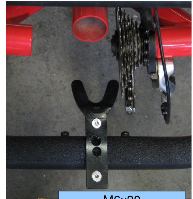
M6x30 Senkkopfschrauben
